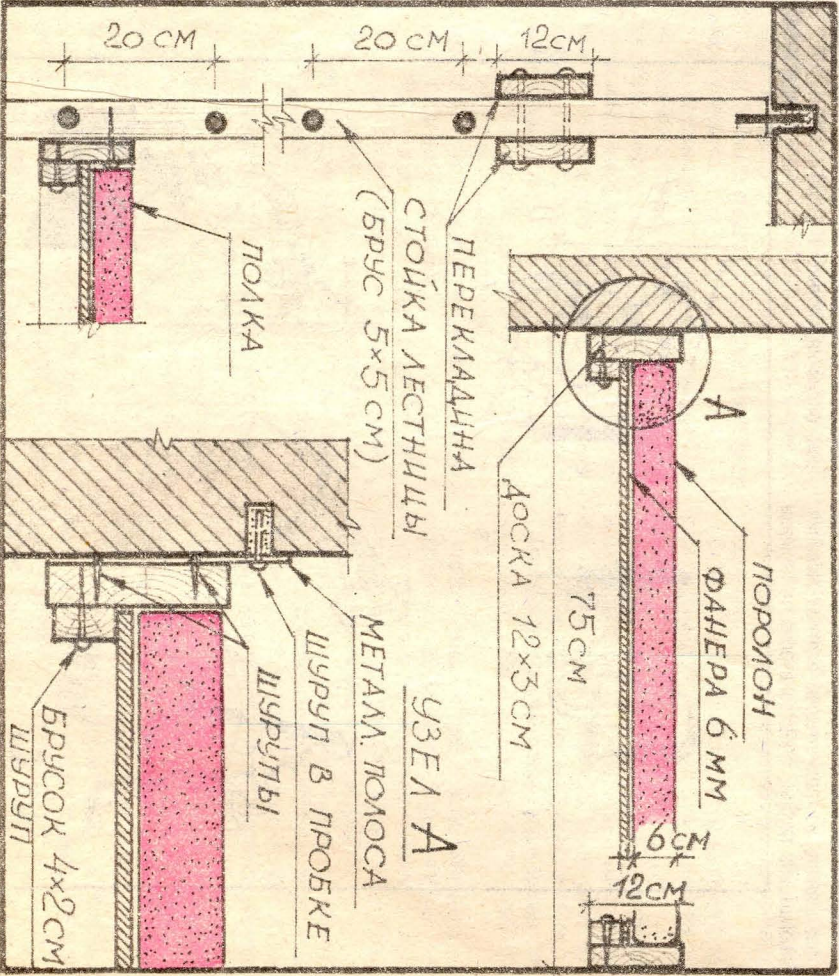
Рис. 2. Детали, узлы.
